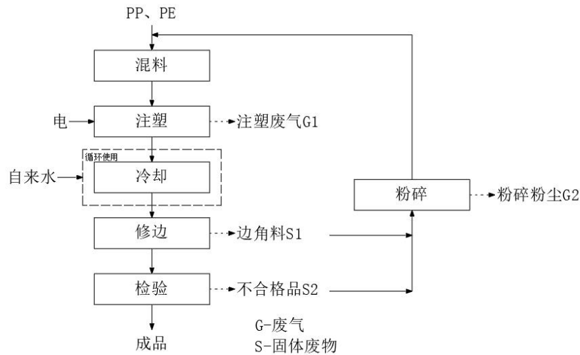
图 2.2-1 变压器配件制造工艺流程及产污环节图
